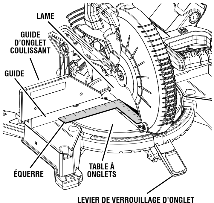
VUE DE LA LAME PAS D'ÉQUERRE AVEC LE GUIDE, DES RÉGLAGES SONT NÉCESSAIRES
