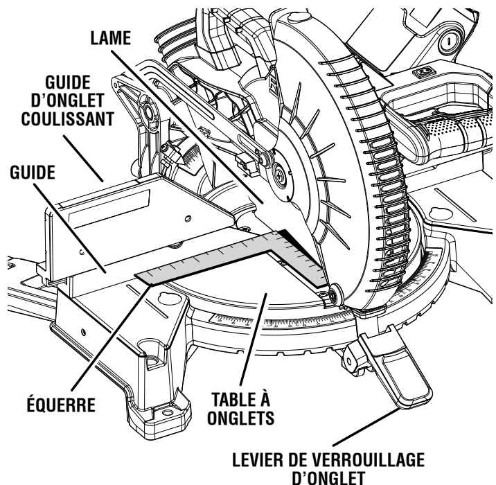
VUE DE LA LAME PAS D'ÉQUERRE AVEC LE GUIDE, DES RÉGLAGES SONT NÉCESSAIRES
