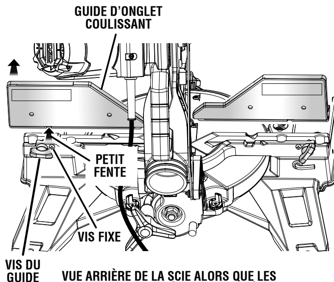
MOULURE COURONNÉE EMBOÎTÉE CONTRE LA FACE DU GUIDE D'ONGLET
