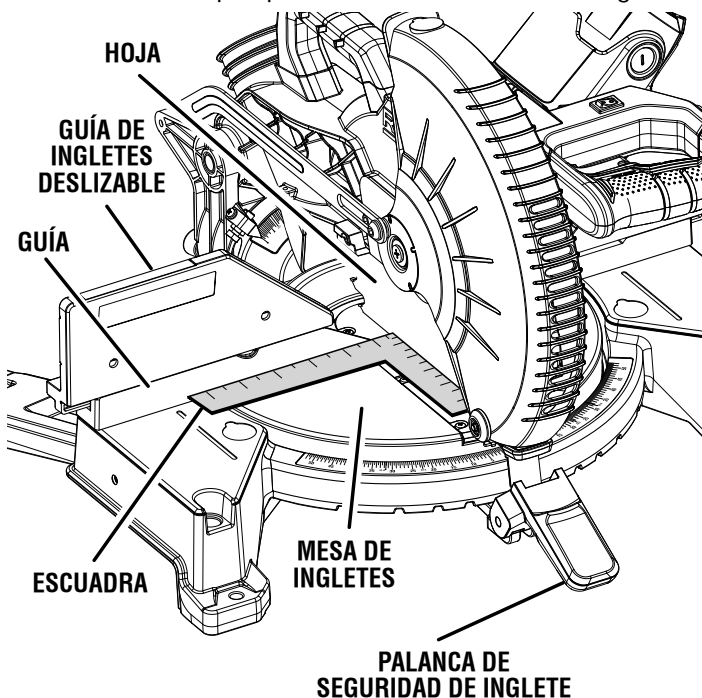
VISTA A DE LA HOJA A ESCUADRA CON LA GUÍA
