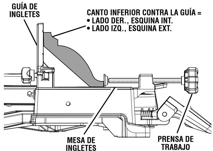
ENCAJE DE MOLDURA DE CORONA GRANDE CONTRA MESA DE INGLETES AL FRENTE TRASERO
