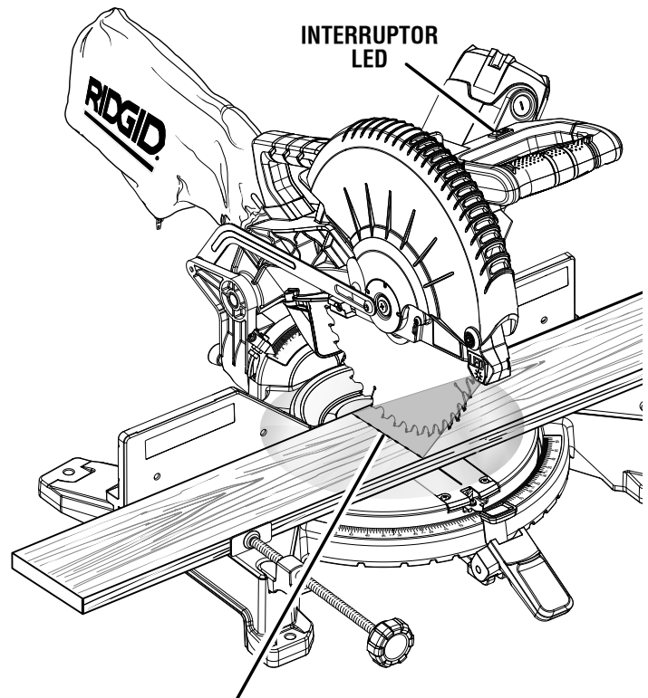
SOMBRA DEL DIENTE DE LA HOJA PROYECTADA EN LA PIEZA DE TRABAJO
