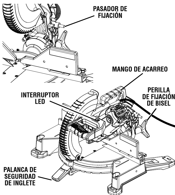
BRAZO DE LA SIERRA ASEGURADO EN LA POSICIÓN INFERIOR
