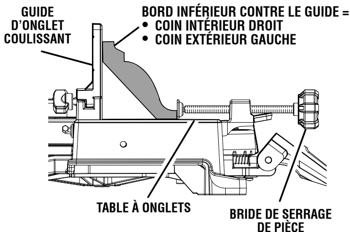
MOULURE COURONNÉE EMBOÎTÉE CONTRE LA FACE DU GUIDE D'ONGLET
