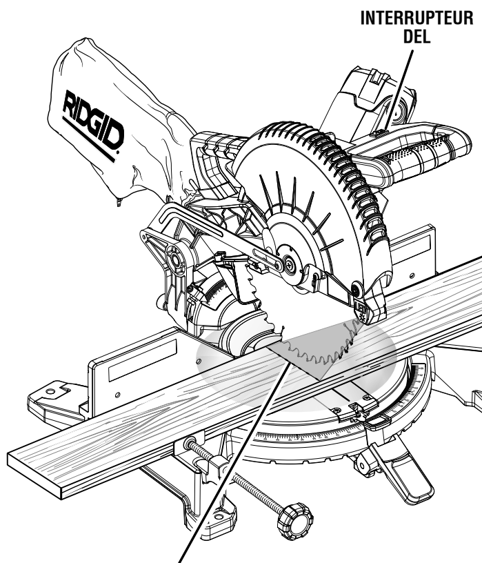
OMBRE DES DENTS DE LA LAME REFLÉTÉE SUR LA PIÈCE À TRAVAILLER
