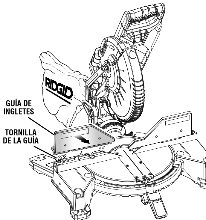
VISTA DE LA SIERRA DESDE ATRÁS CON LAS GUÍAS MIRANDO HACIA ADELANTE
