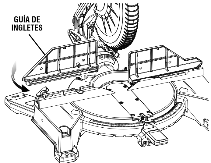
VISTA DE LA SIERRA DESDE EL FRENTE CON LAS GUÍAS MIRANDO HACIA ATRÁS
