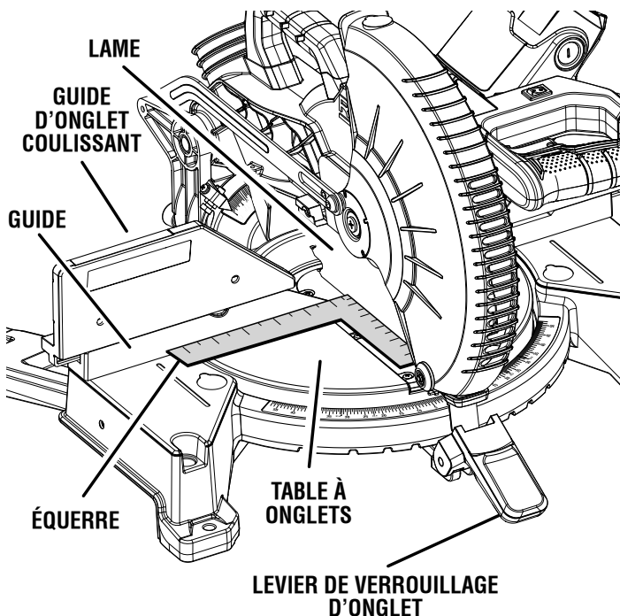
VUE DE LA LAME D'ÉQUERRE AVEC LE GUIDE
