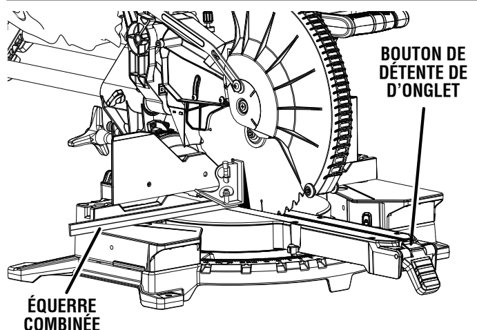
VUE DE LA LAME PAS D'ÉQUERRE AVEC LA TABLE, DES RÉGLAGES SONT NÉCESSAIRES
