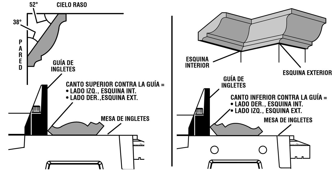
MOLDURA DE CORONA EN POSICIÓN HORIZONTAL EN LA MESA DE INGLETES
