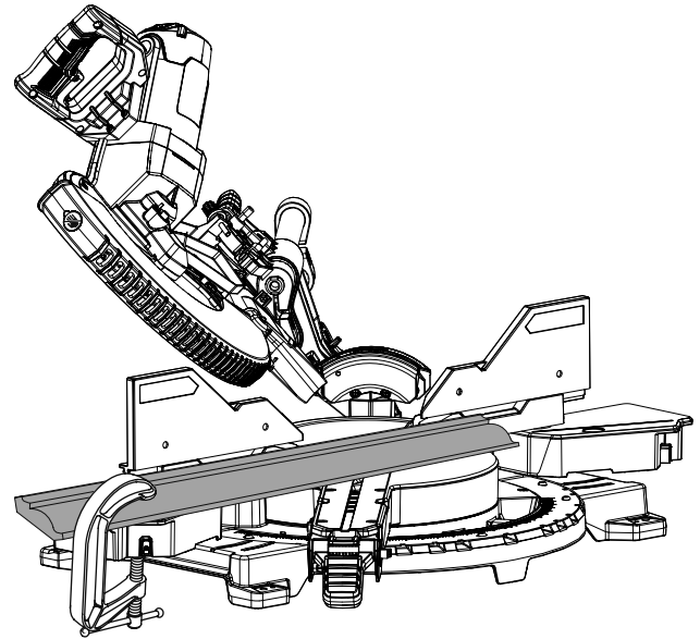
45° x 45° CORTE EN BISEL COMBINADO
